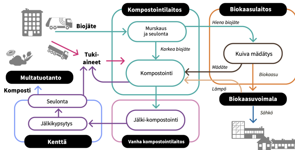
Biojätteen käsittelyn yleiskuva (kuiva osavirtamädätys)
